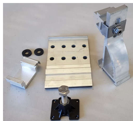
seitliche Montage (horiz., höhenverst. + starr)
